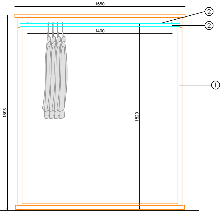
SECCION
