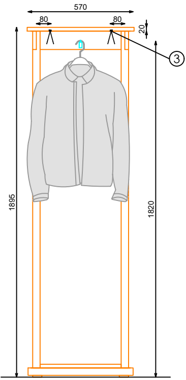
SECCION
