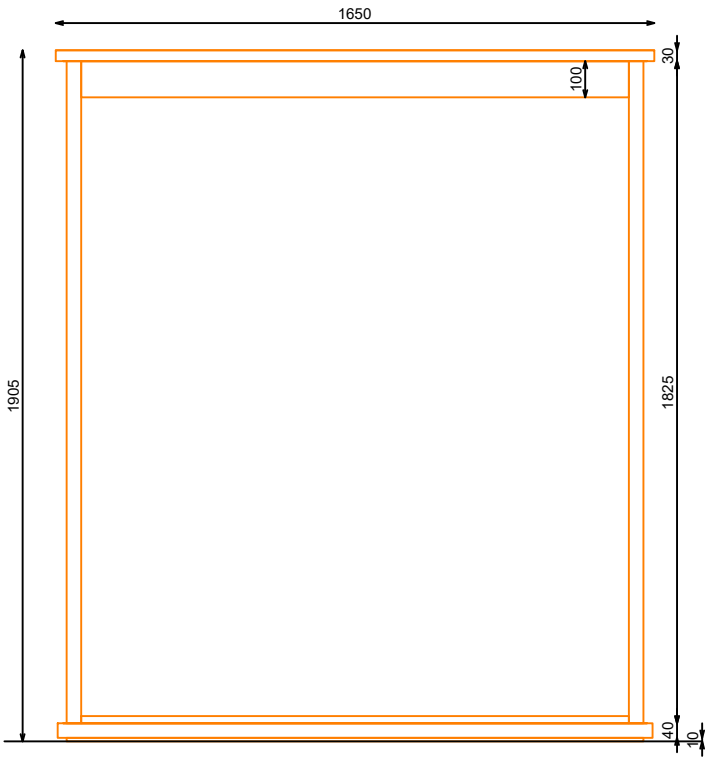
ALZADO
