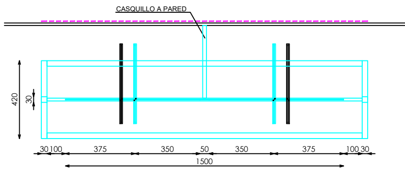
PLANTA
