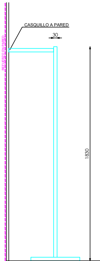
ALZADO LATERAL
