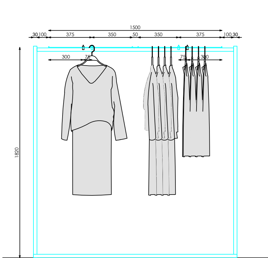
ALZADO
