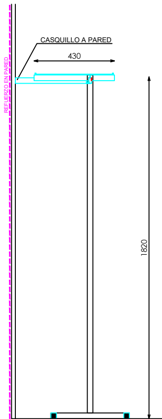
SECCIÓN
