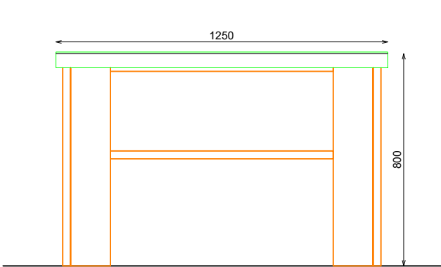
ALZADO FRONTAL
