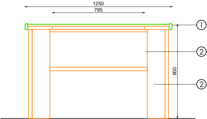
ALZADO LATERAL
