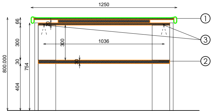
SECCION
