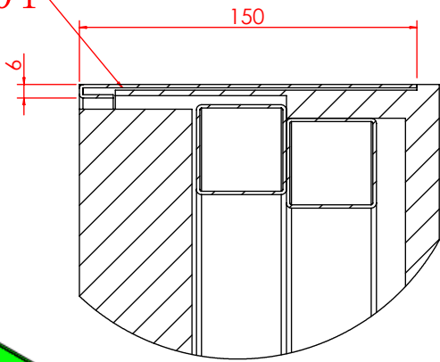
局部视图 AJ 比例 1:3
