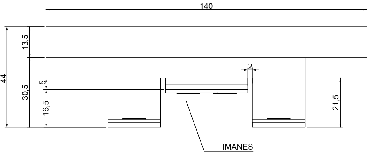
PLANTA
