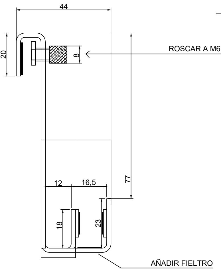
PERFIL
