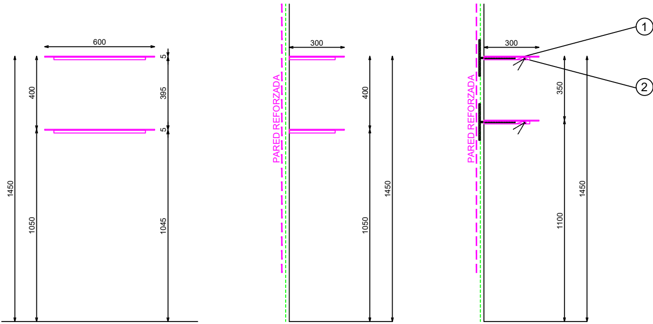
ALZADO
