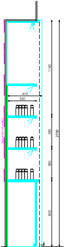
SECCION
