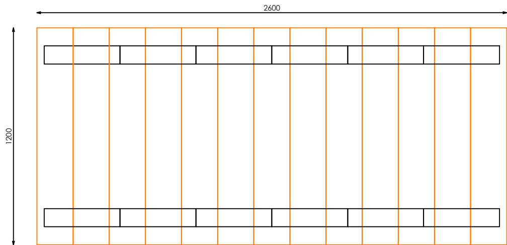
PLANTA
