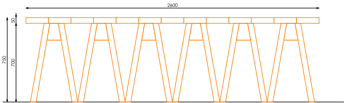
ALZADO FRONTAL
