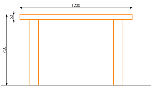
ALZADO LATERAL
