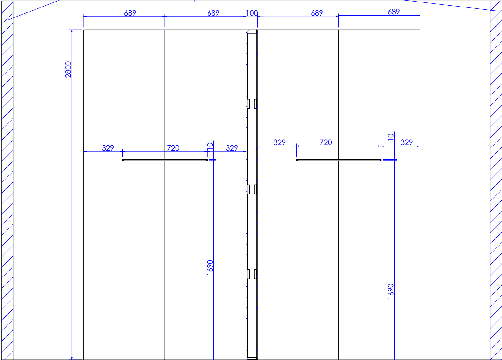
剖面 AJ-AJ
