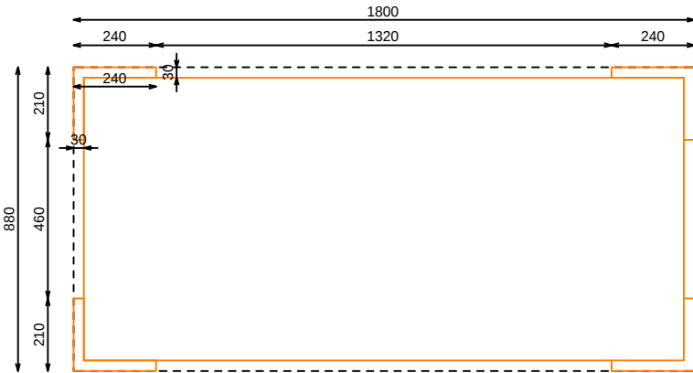
PLANTA (PATAS)
