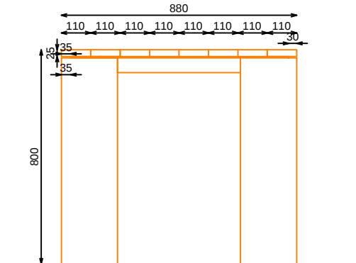
PERFIL
