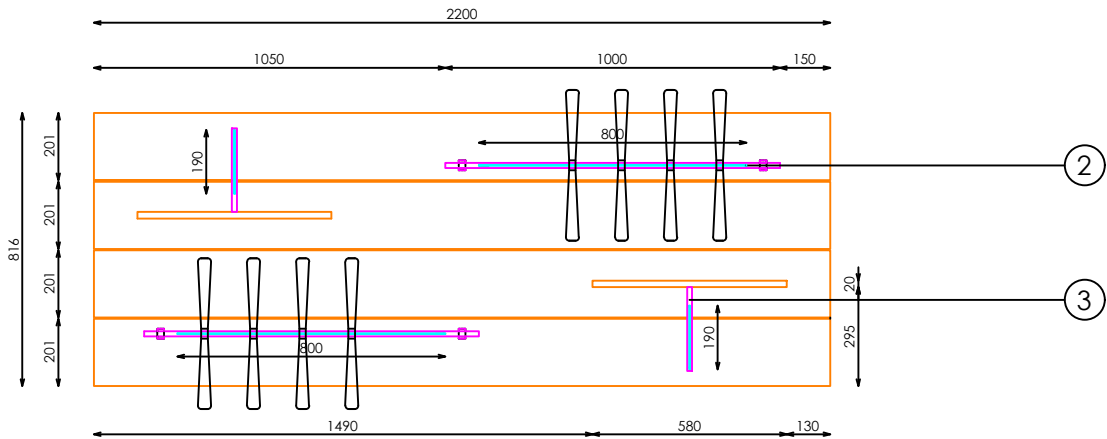
PLANTA
