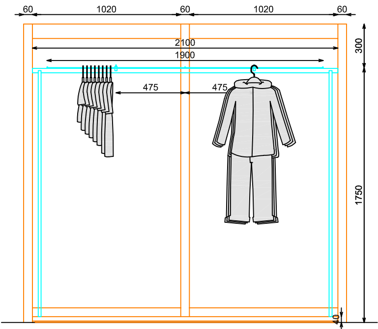
ALZADO FRONTAL
