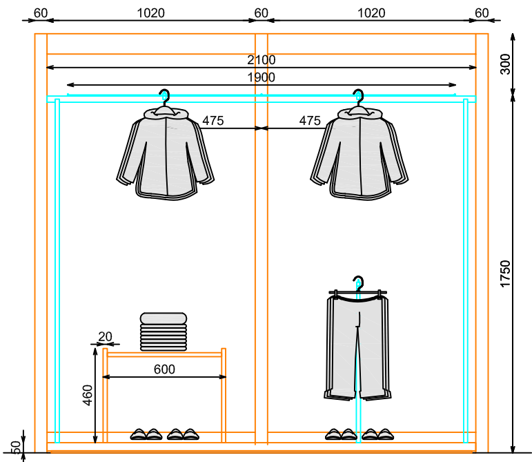
ALZADO TRASERO
