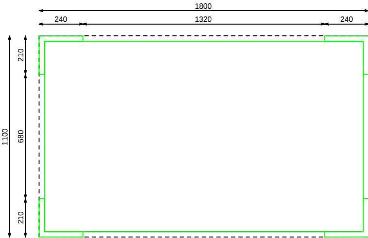
PLANTA (PATAS)
