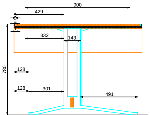
SECCION
