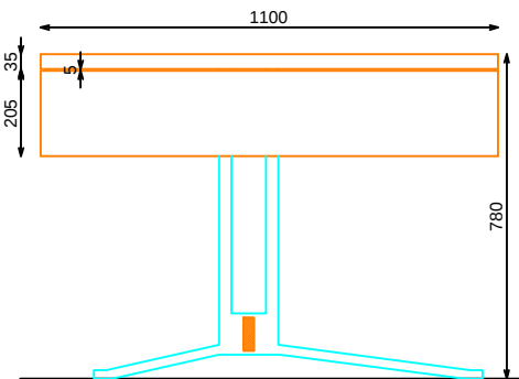
ALZADO LATERAL
