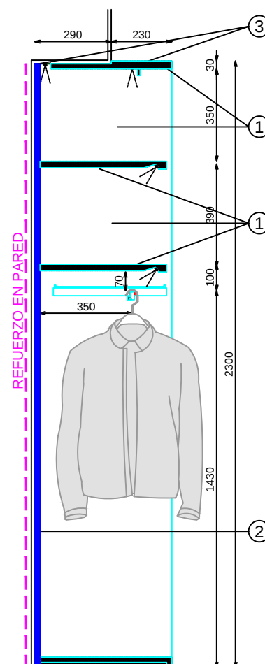
SECCION BARRA BAJA
