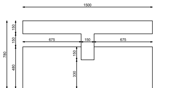
ALZADO FRONTAL
