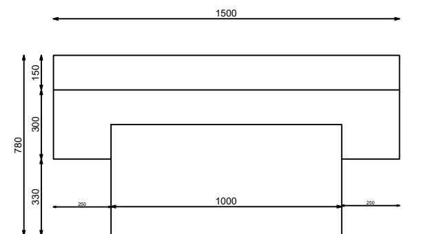
ALZADO LATERAL
