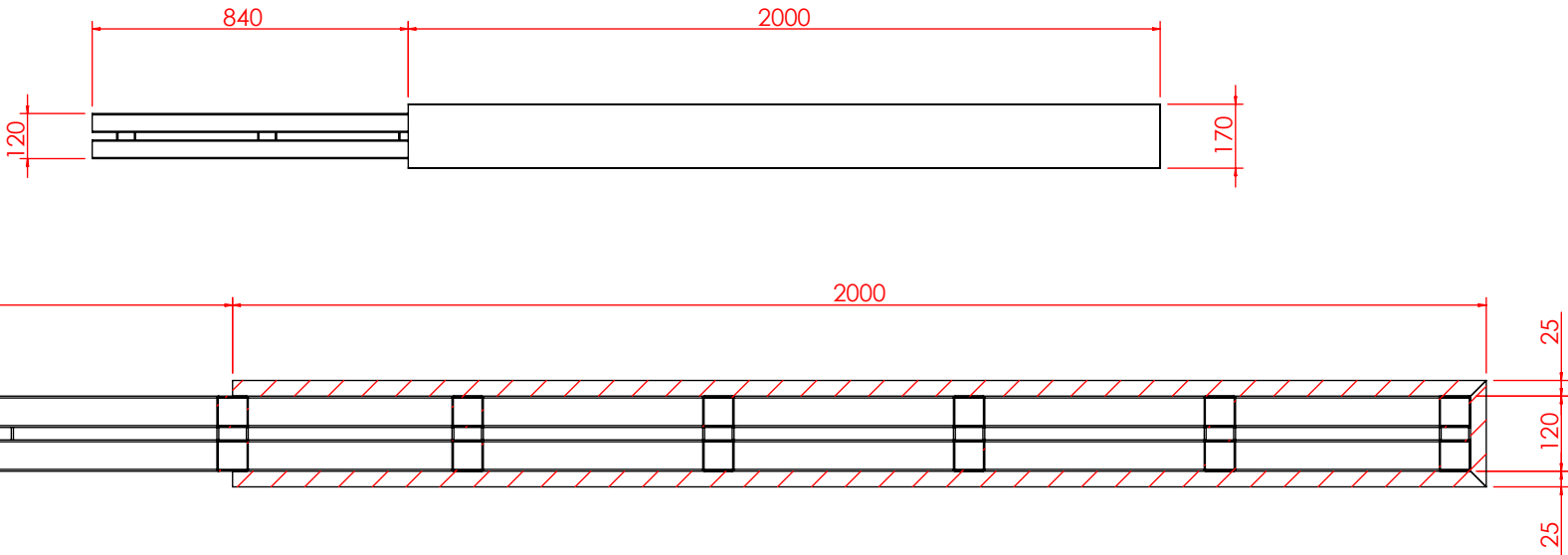
剖面 AH-AH 比例 1 : 12
