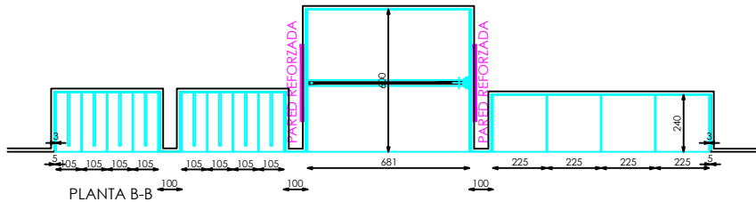
PLANTA B-B
