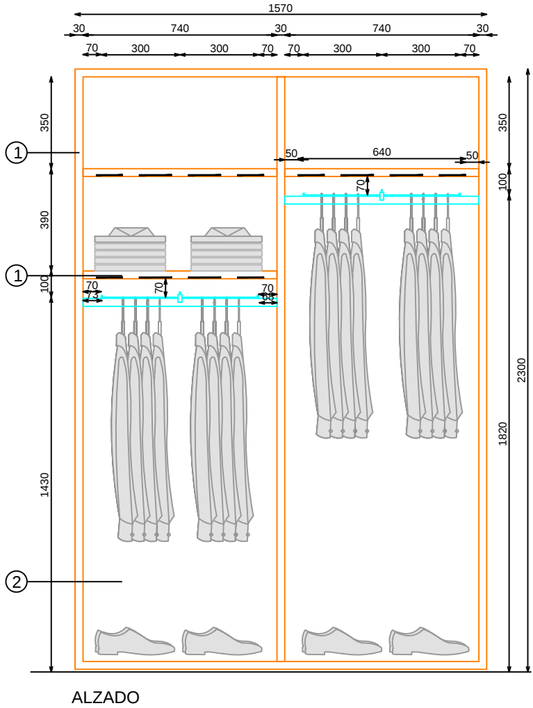
ALZADO
