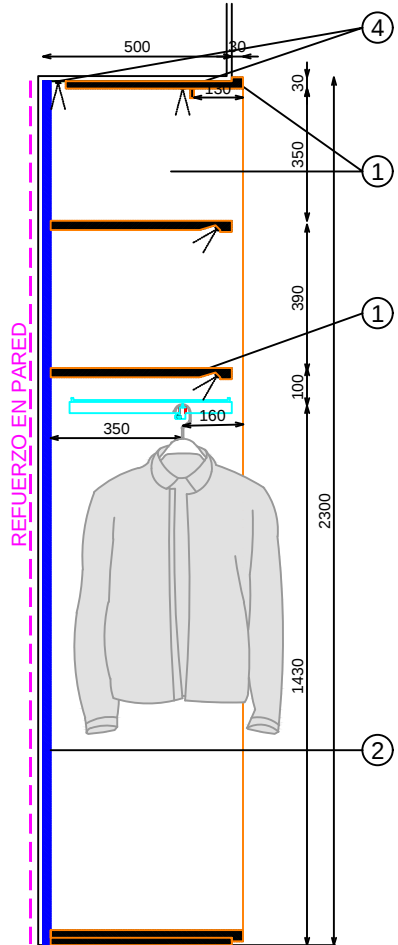
SECCION BARRA BAJA
