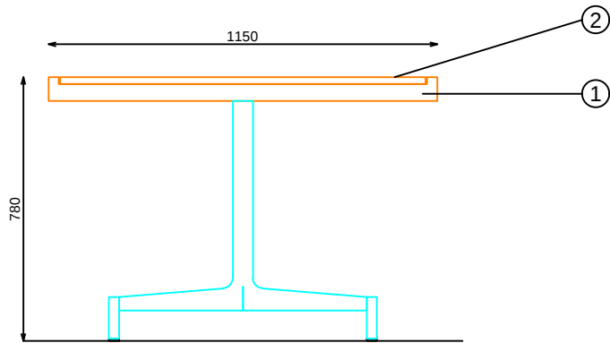
SECCION
