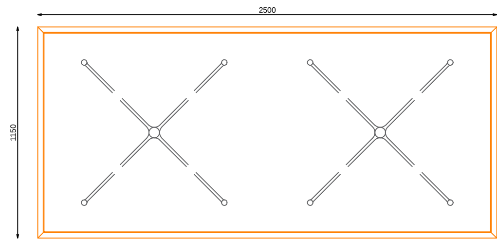
PLANTA
