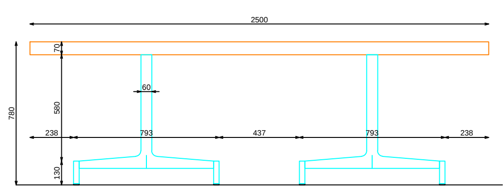
ALZADO FRONTAL
