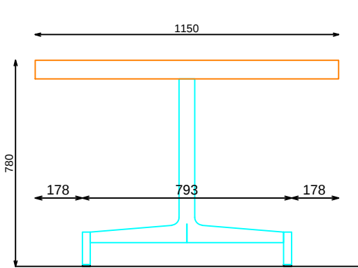
ALZADO LATERAL
