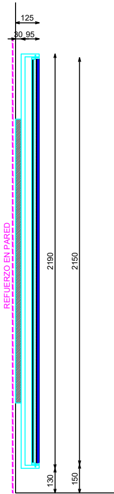
SECCION
