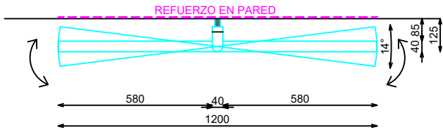
PLANTA
