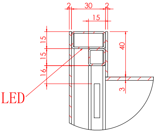
局部视图 AH 比例 1:2
