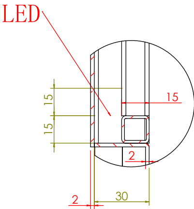
局部视图 AJ 比例 1:2
