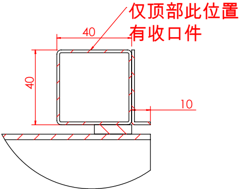
局部视图 AJ 比例 1:2
