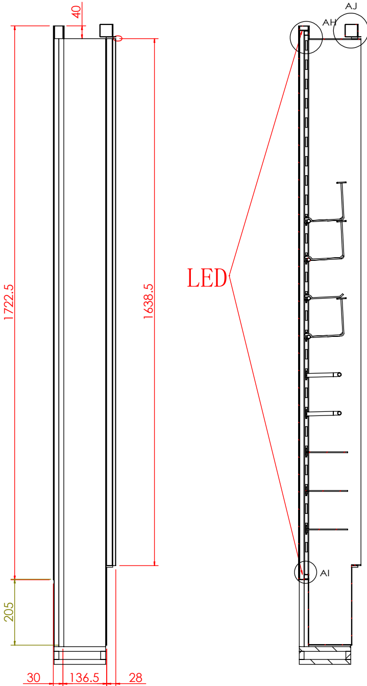
剖面 AG-AG
