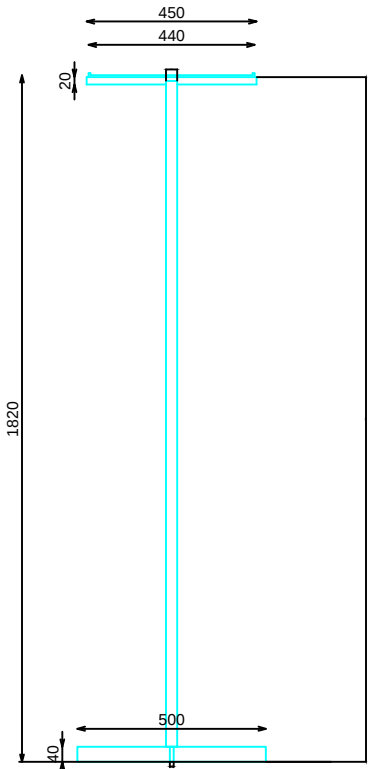
ALZADO
