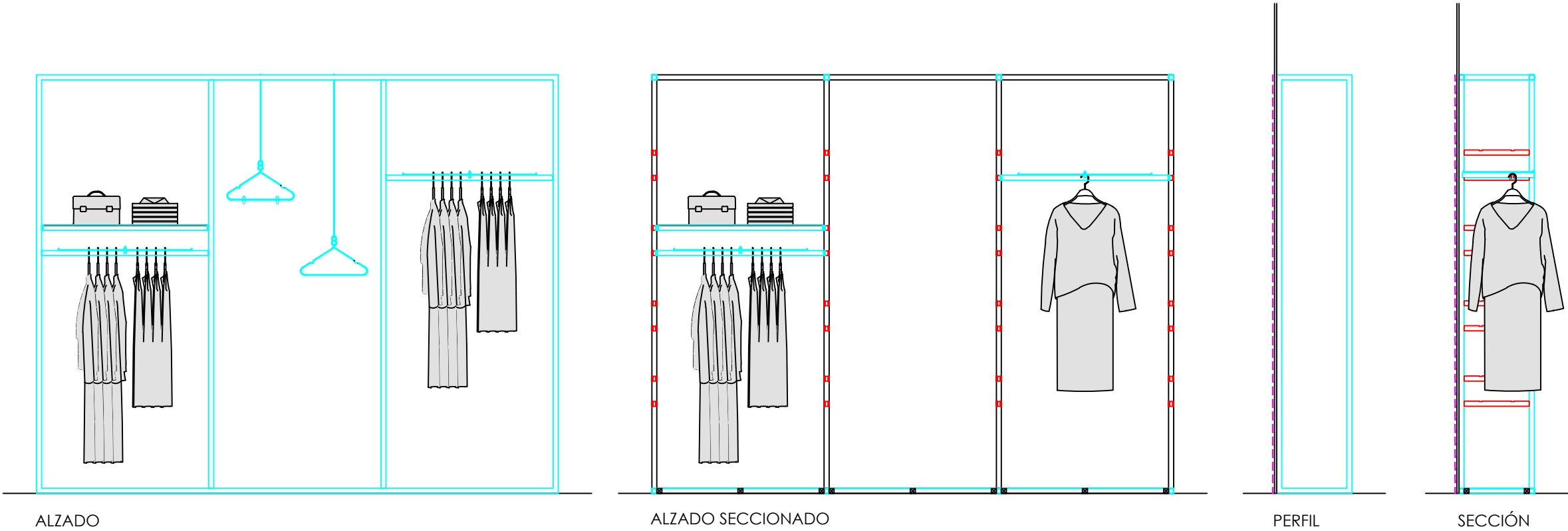
ALZADO
