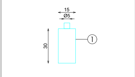
DETALLE BARRA
