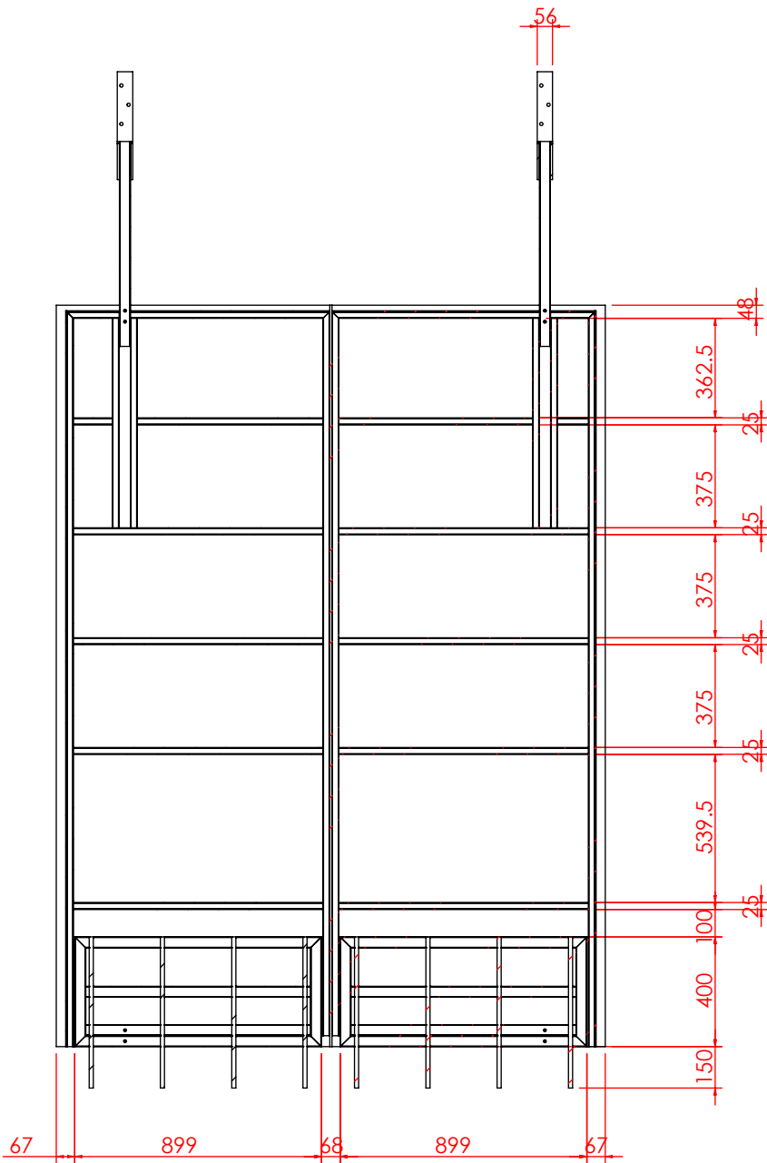
剖面 AG-AG
