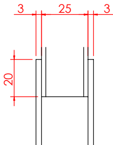
局部视图 AH 比例 1:2
