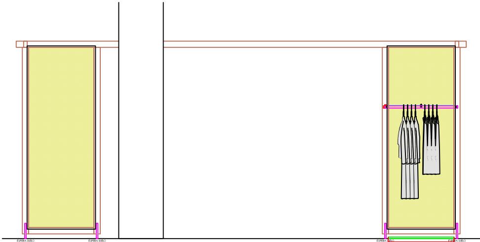
ALZADO FRONTAL
