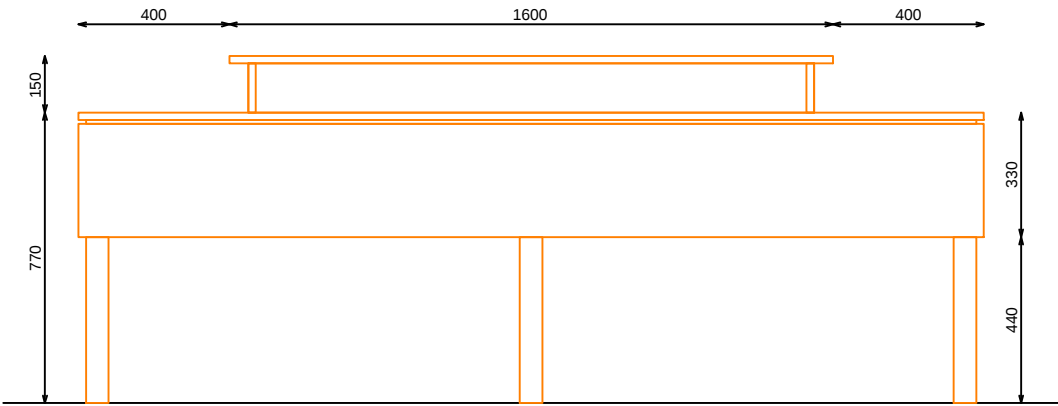
ALZADO
