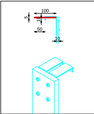
BALDA PLANA PAQUETERIA 420x400
