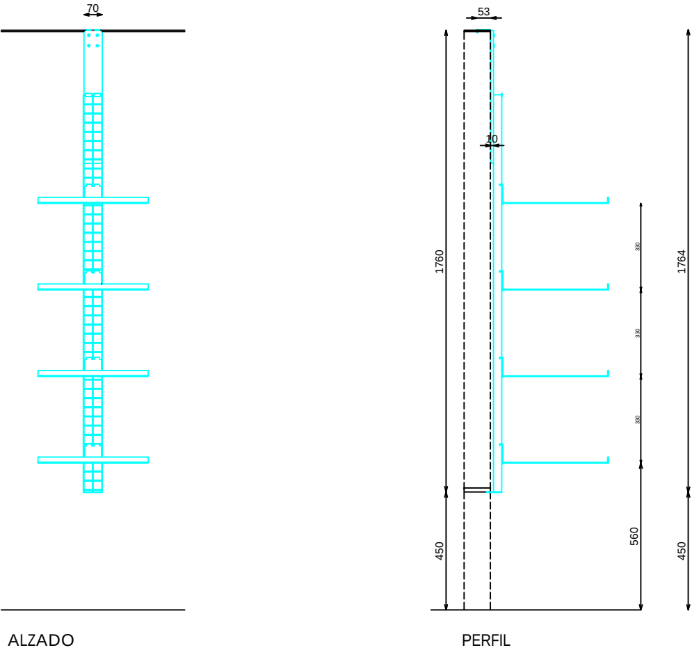
ALZADO
