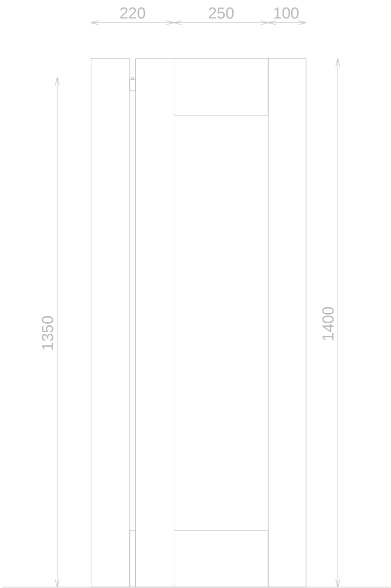
ALZADO DERECHO
