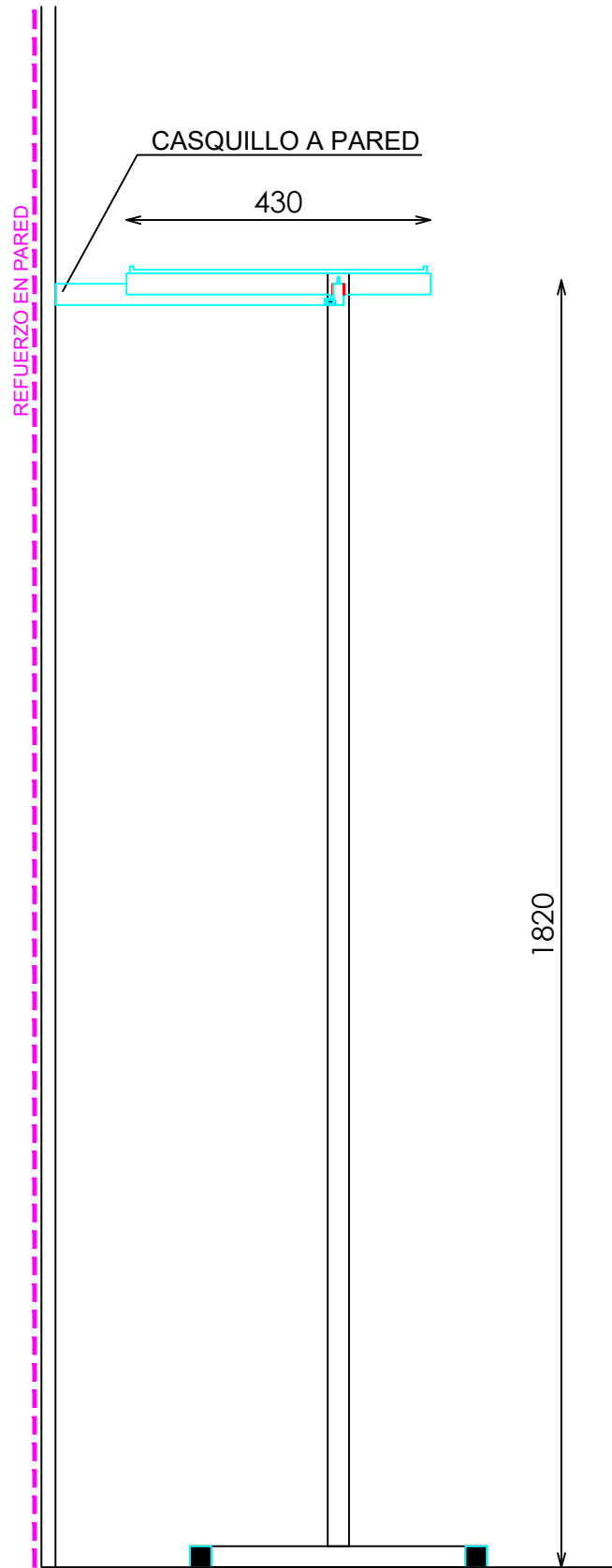
SECCIÓN
