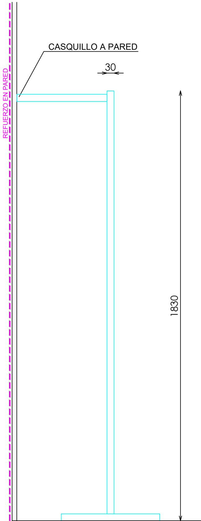
ALZADO LATERAL
