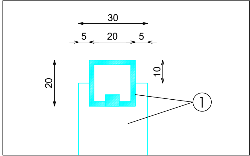
DETALLE B
