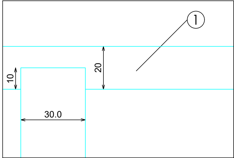
DETALLE C
