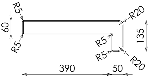
ALZADO LATERAL
