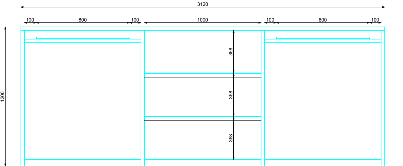
ALZADO
