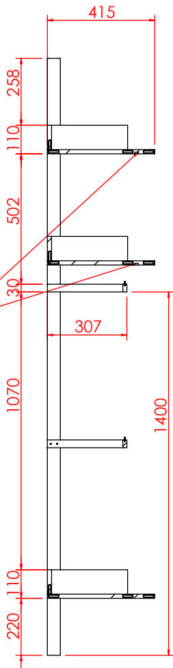
剖面 AH-AH
