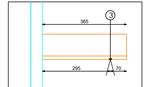
DETALLE ESTANTE MODULO PQ/BAS
