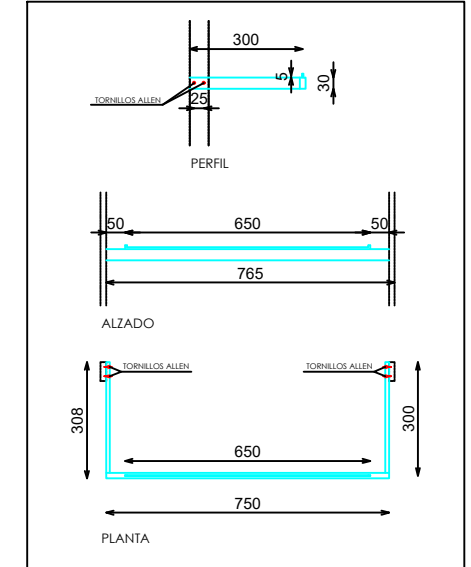
DETALLE ESTANTE MODULO INT
