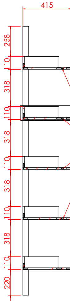
剖面 AG-AG
