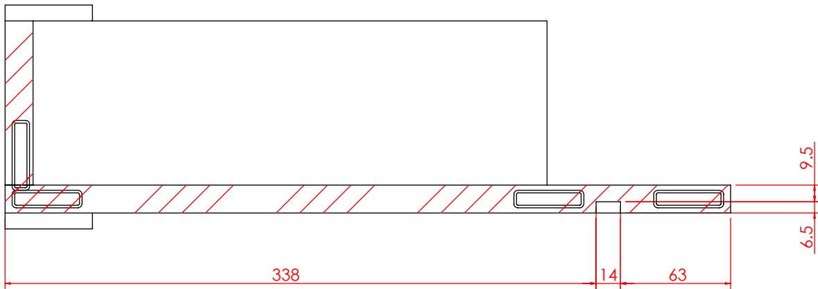
剖面 AG-AG
