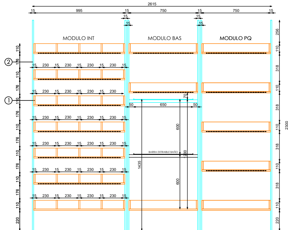
ALZADO FRONTAL
