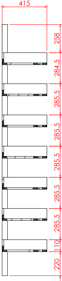
剖面 AK-AK
