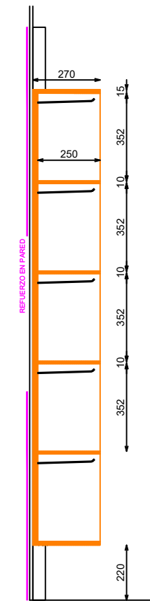
PERFIL MODULO CALC
