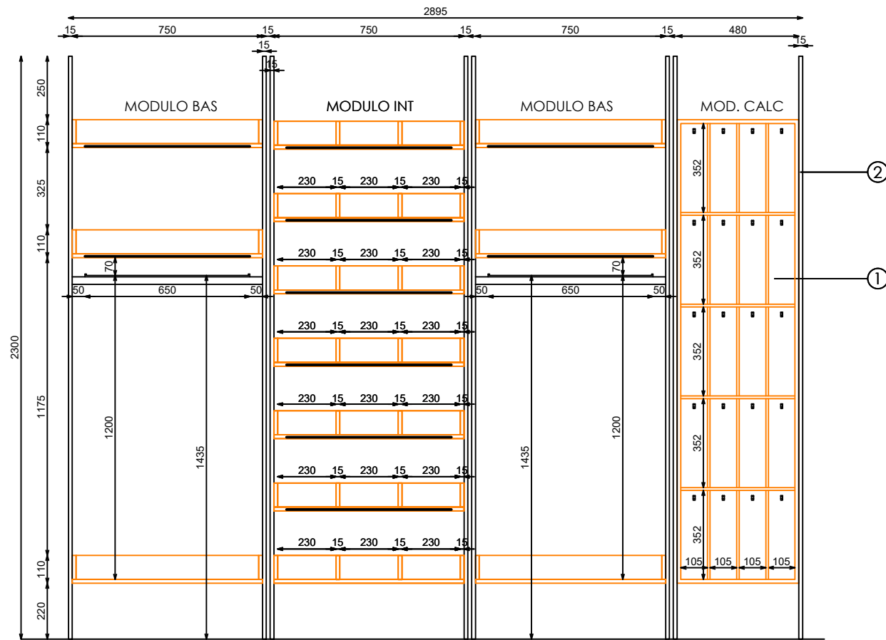
ALZADO FRONTAL
