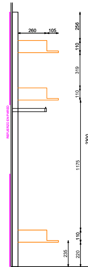
PERFIL MODULO BAS
