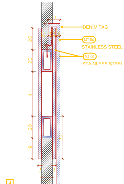
4 1:1 DETAIL
