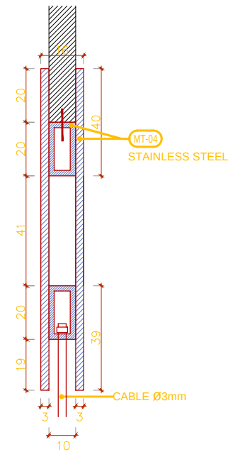
5 1:1 DETAIL
