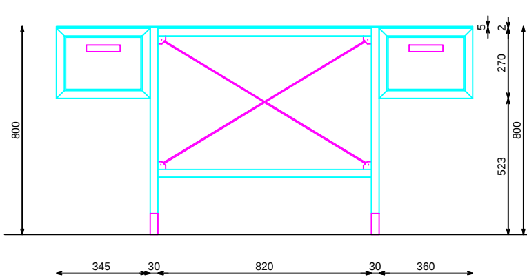
ALZADO FRONTAL
