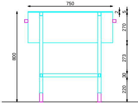
SECCION
