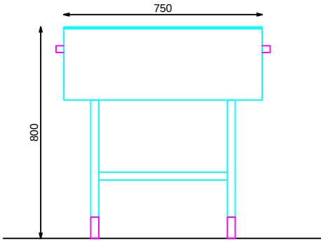
ALZADO LATERAL
