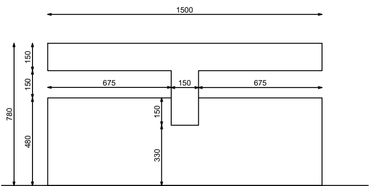
ALZADO FRONTAL
