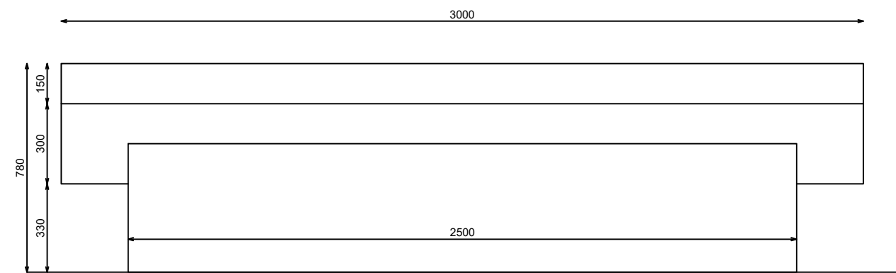
ALZADO LATERAL
