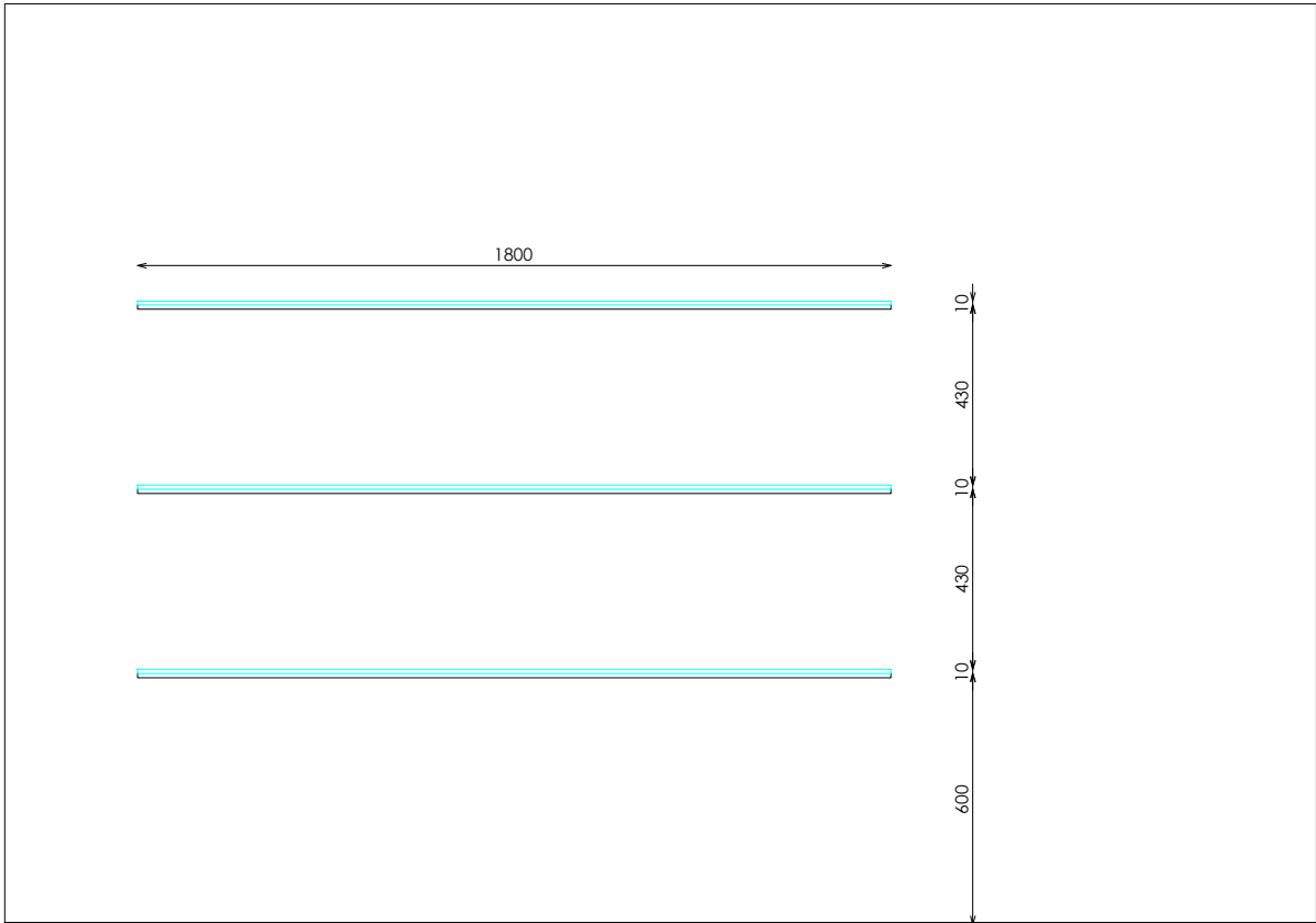
ALZADO
