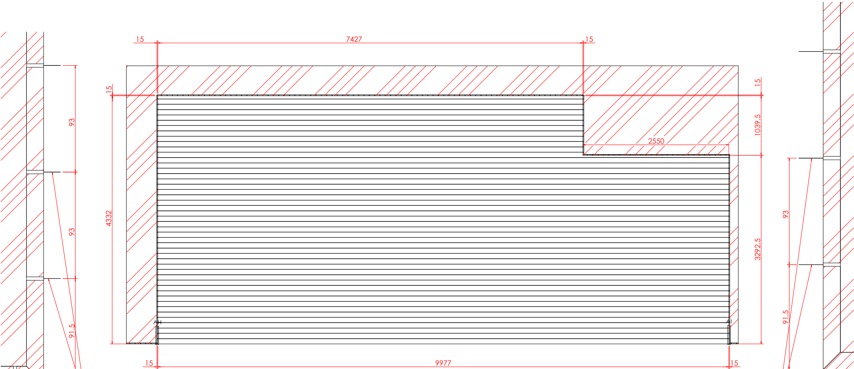
俯视图 地板拼缝和墙板的拼缝 居中对齐 地板拼缝和墙板的拼缝 居中对齐
