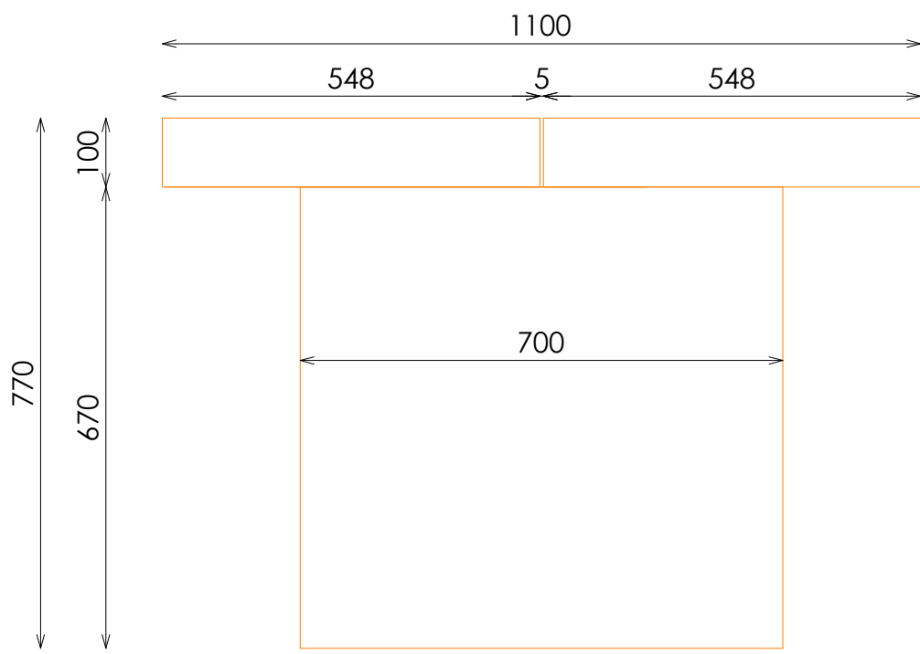
ALZADO LATERAL
