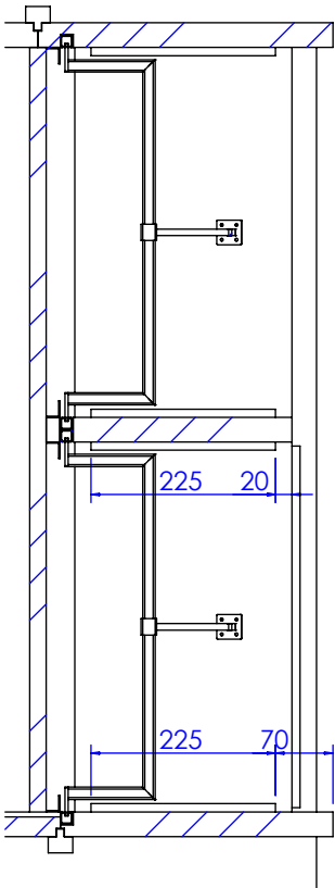
局部视图 AP 比例 1 : 10
