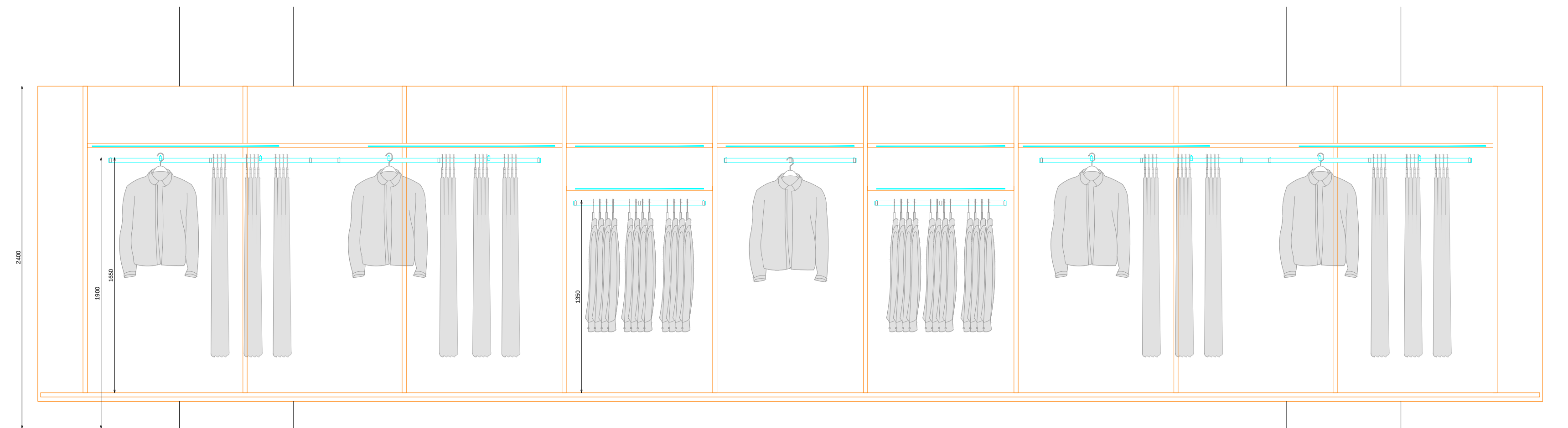
ALZADO
