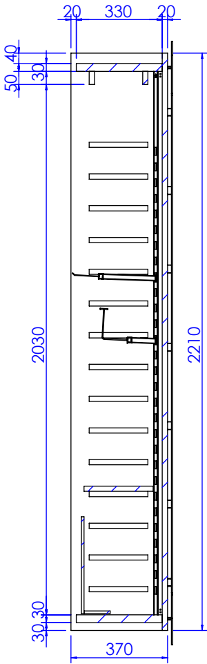
剖面 AG-AG
