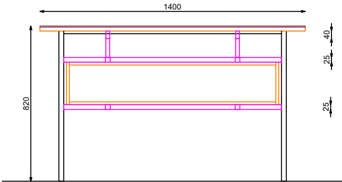
ALZADO LATERAL
