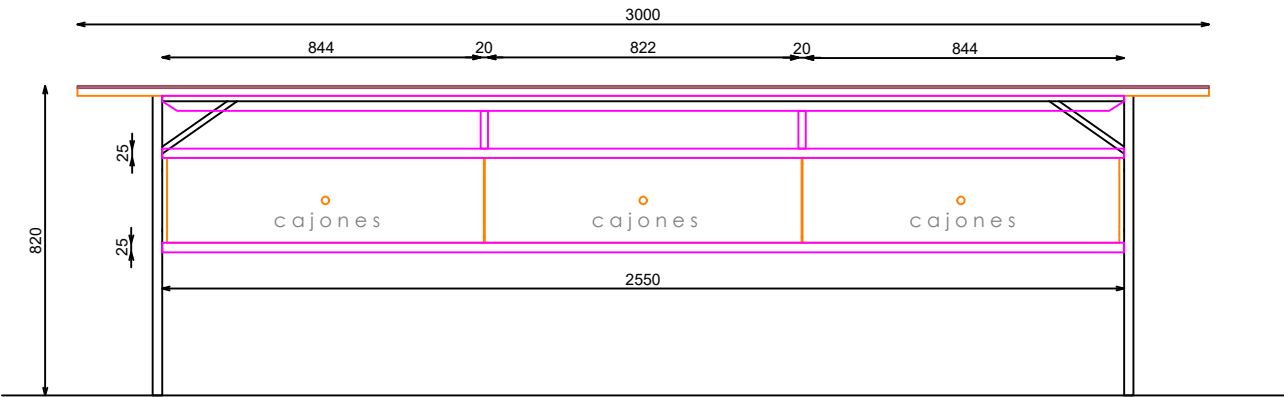
ALZADO FRONTAL
