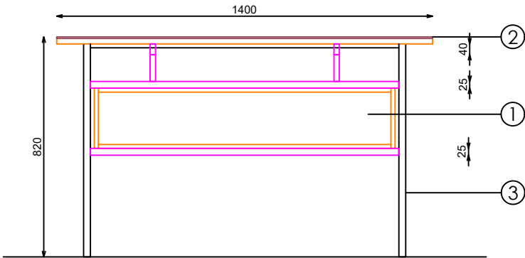
ALZADO LATERAL
