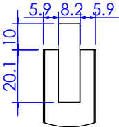
局部视图 AH 比例 1 : 2
