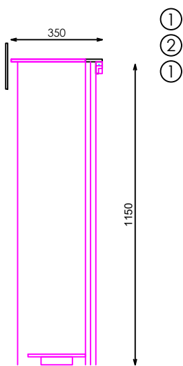
SECCIÓN
