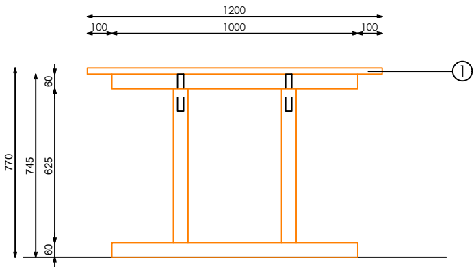
ALZADO LATERAL
