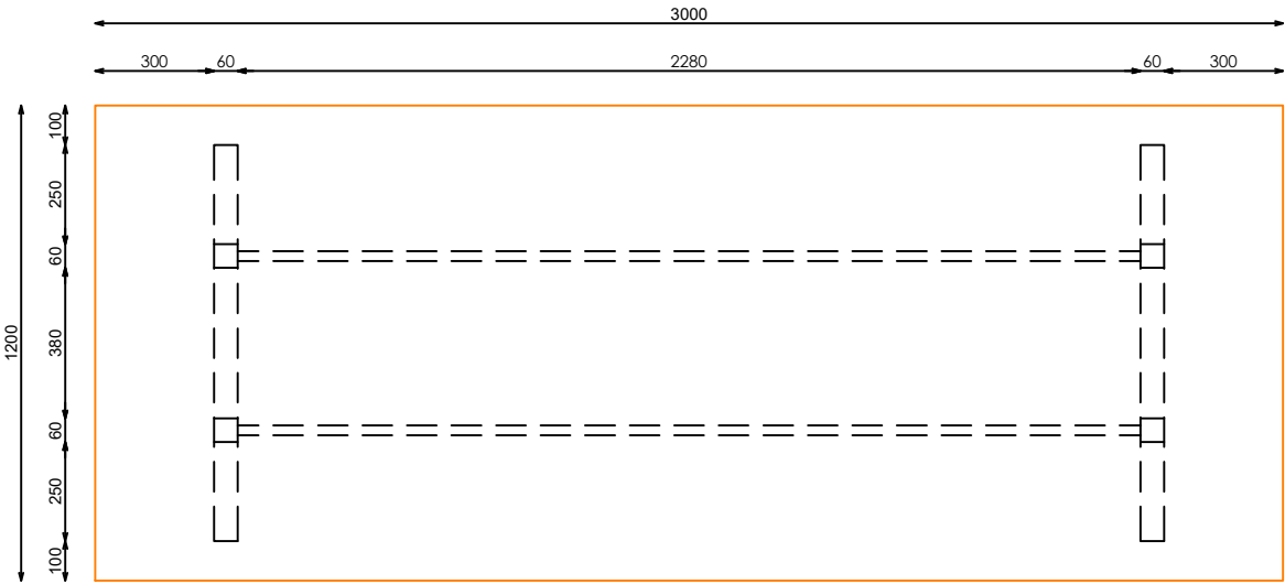
PLANTA SECCIONADA
