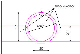
DETALLE D
