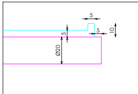
DETALLE C
