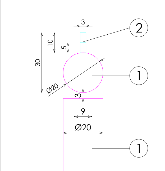
DETALLE ANTIROCE
