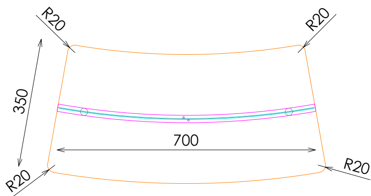
PLANTA
